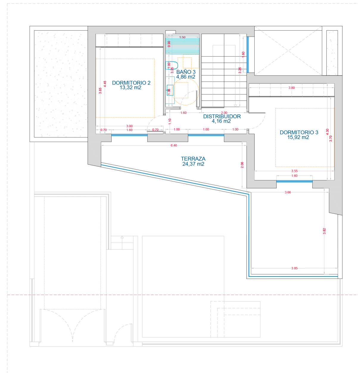
PLANTA PISO
